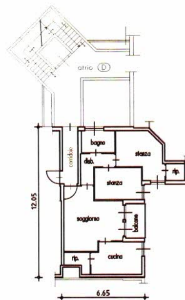
PIANO SECONDO SCALA 1 : 200 - H. 2.60
