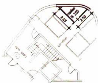
PRIMO SOTTOSTRADA SCALA 1 : 200
